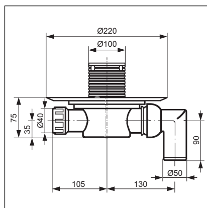
Рис. 7: Чертеж с размерами, модель 4935.3
